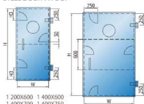
STEEL DOOR TYPE DF
