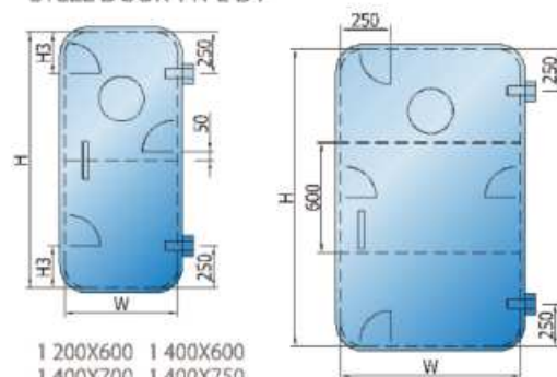
STEEL DOOR TYPE DY
